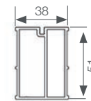
wymiary wysokiego legara aluminiowego (mm)
