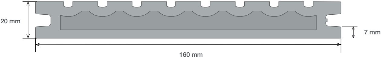
ryflowana strona deski
